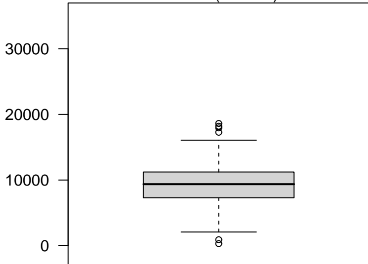
Node 2 (n = 145)
