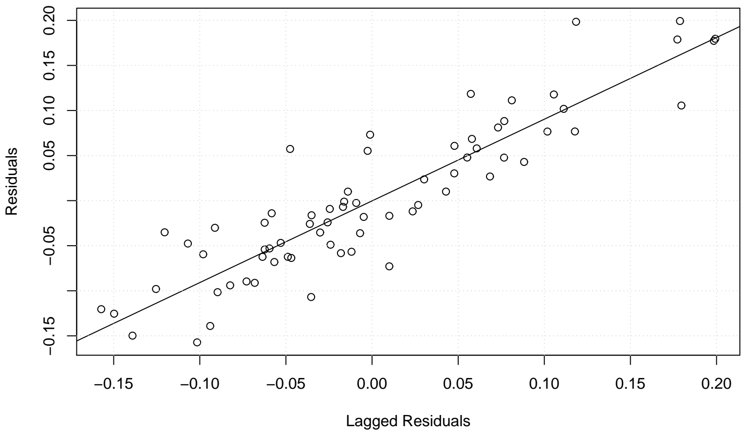
Lag plot
