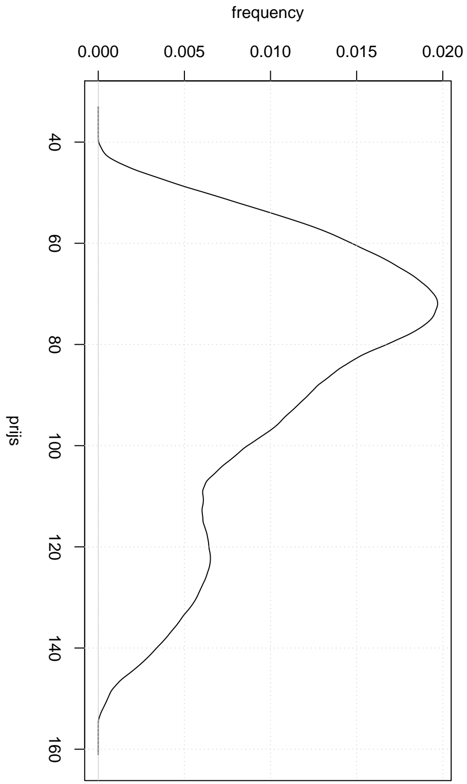
Epanechnikov Kernel
