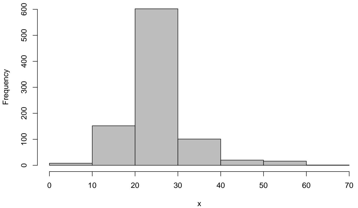
frequentietabel van 6 bins
