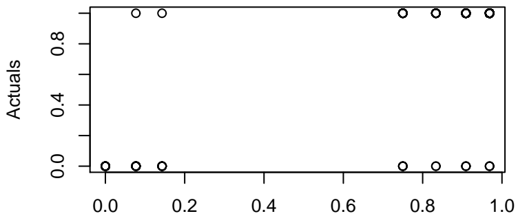
Actuals versus Predictions
