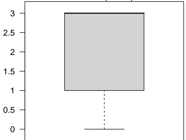
Node 3 (n = 46)
