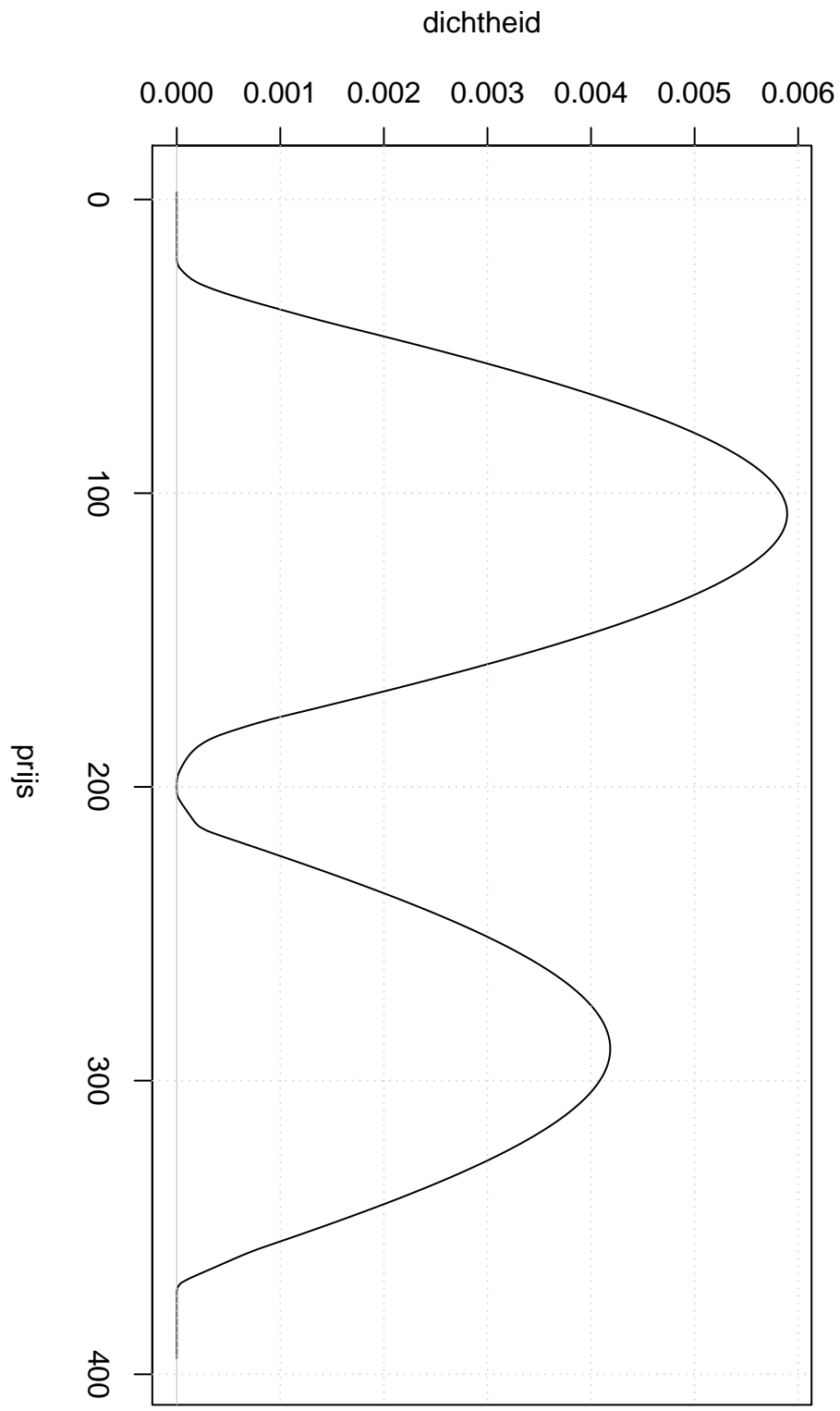
Optcosine Kernel
