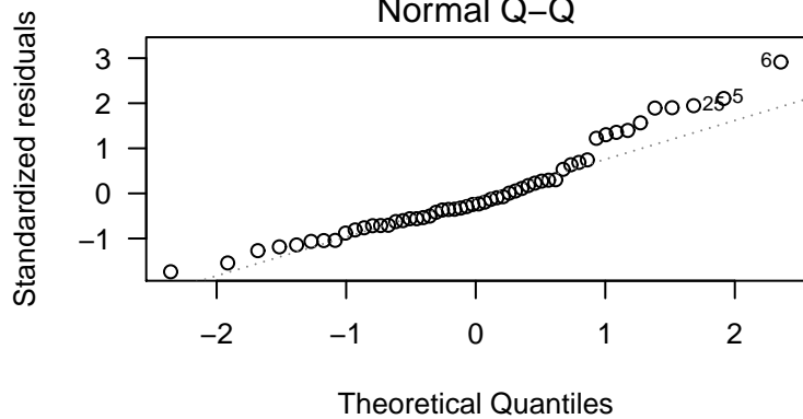
Normal Q-Q
