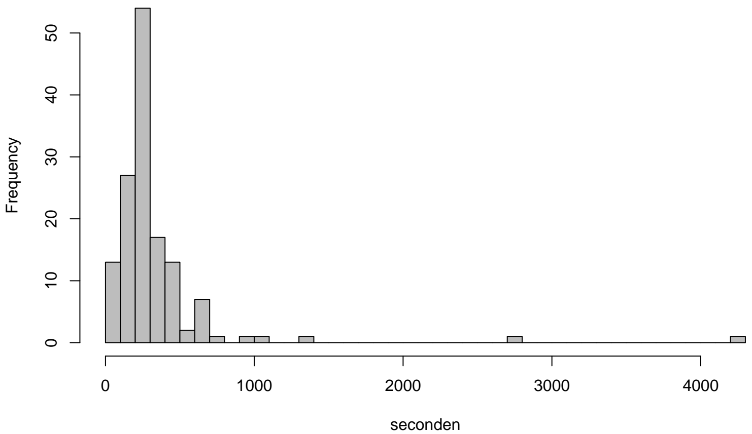
Histogram: Reproductie met 30 klassen
