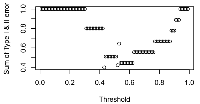
(1-Sens.) + (1-Spec.)
