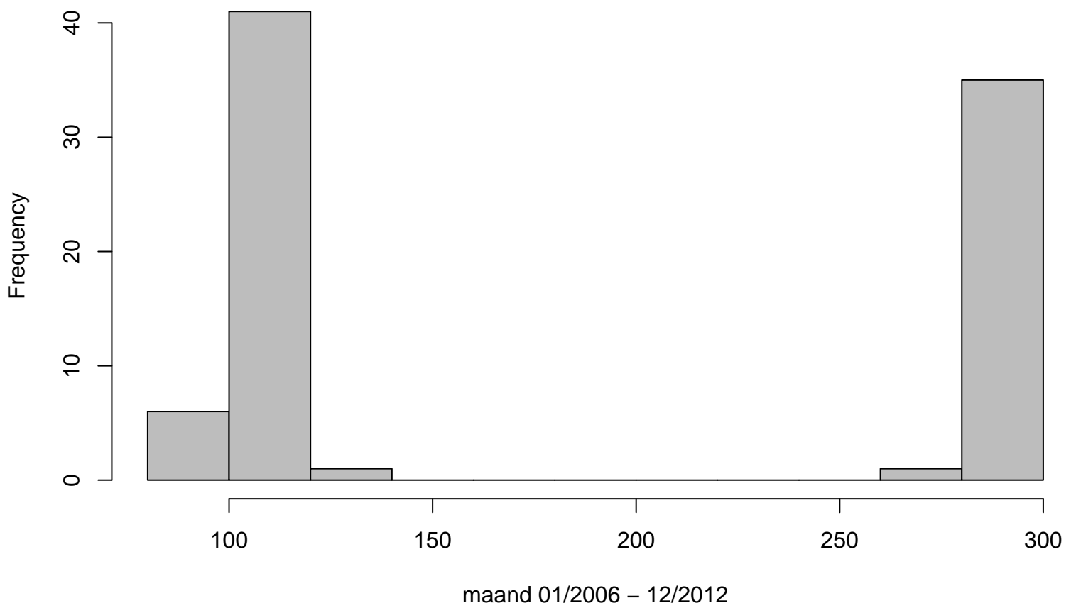
Histogram gem. consumptieprijzen GSM
