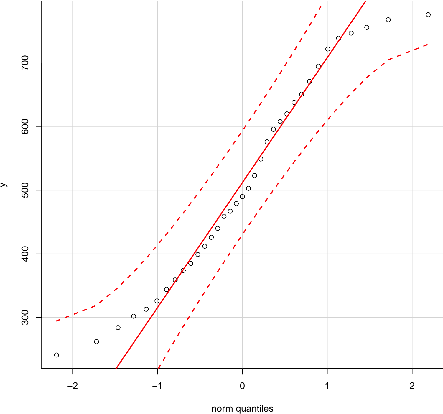
QQplot of variable y
