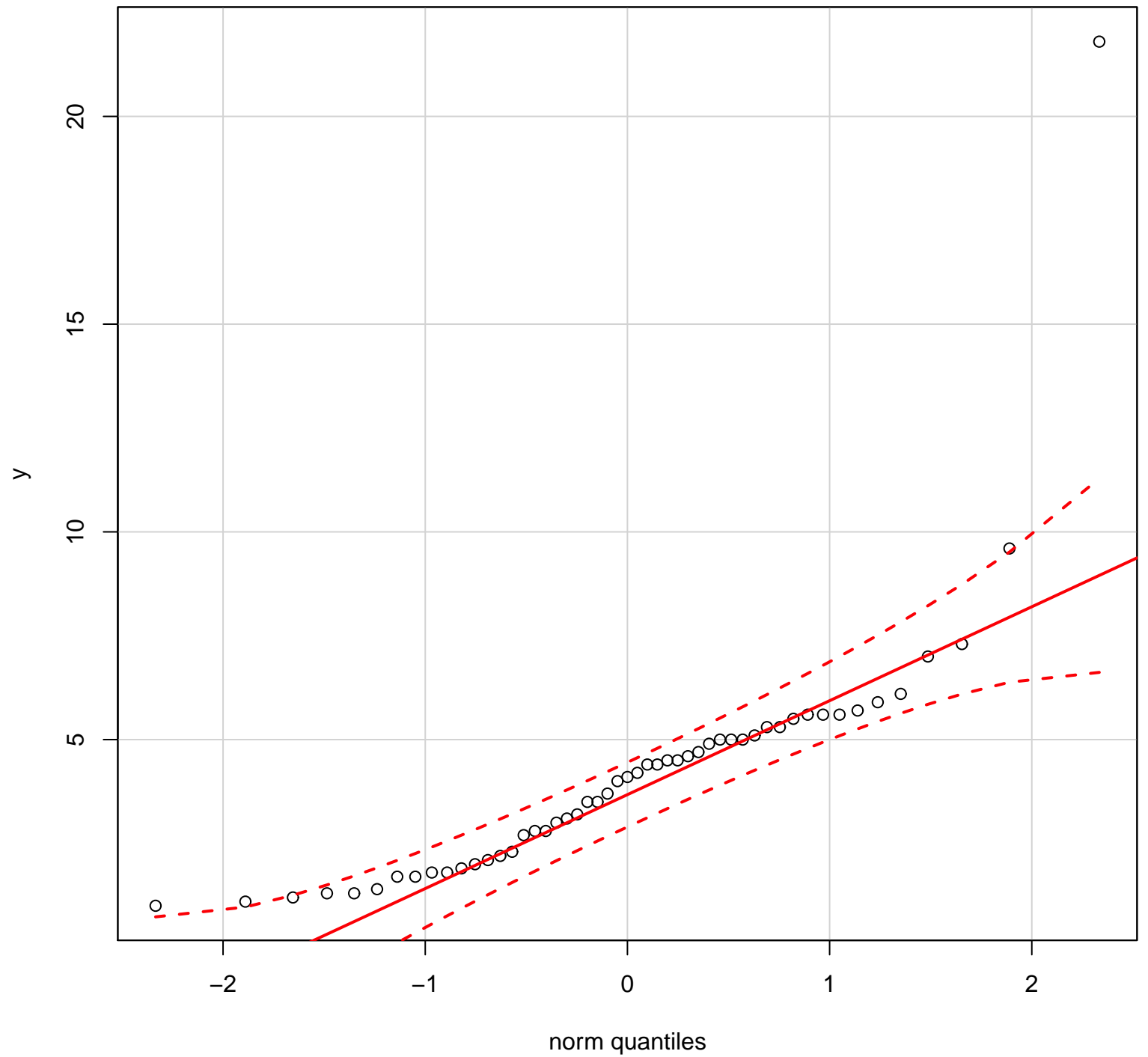
QQplot of variable y
