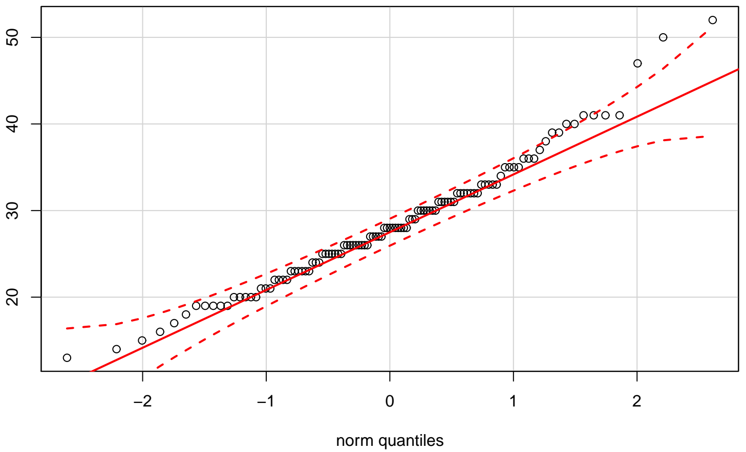
QQplot of variable y
