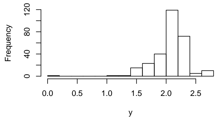
Histogram of y
