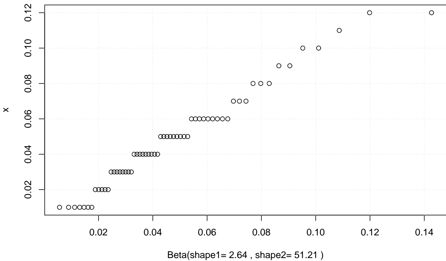
QQ plot (Beta)
