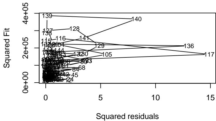
Sq.Resid vs. Sq.Fit
