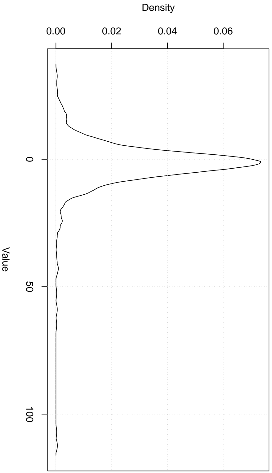
Epanechnikov Kernel
