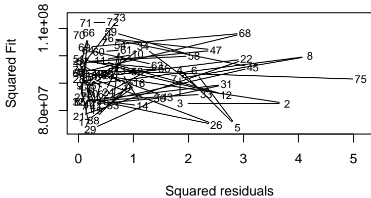
Sq.Resid vs. Sq.Fit
