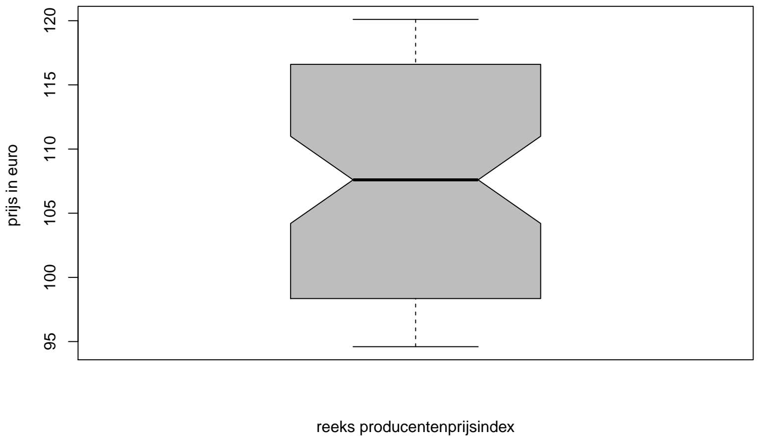
boxplot producentenprijsindex
