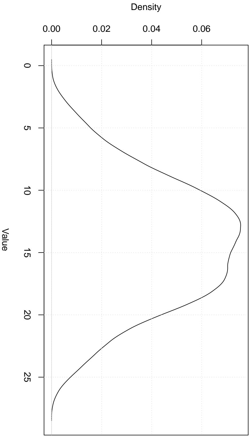
Cosine Kernel
