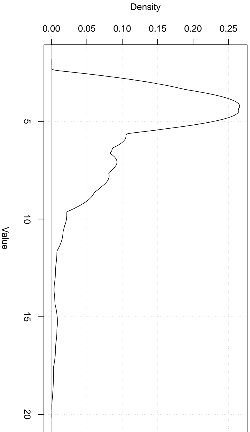
Epanechnikov Kernel
