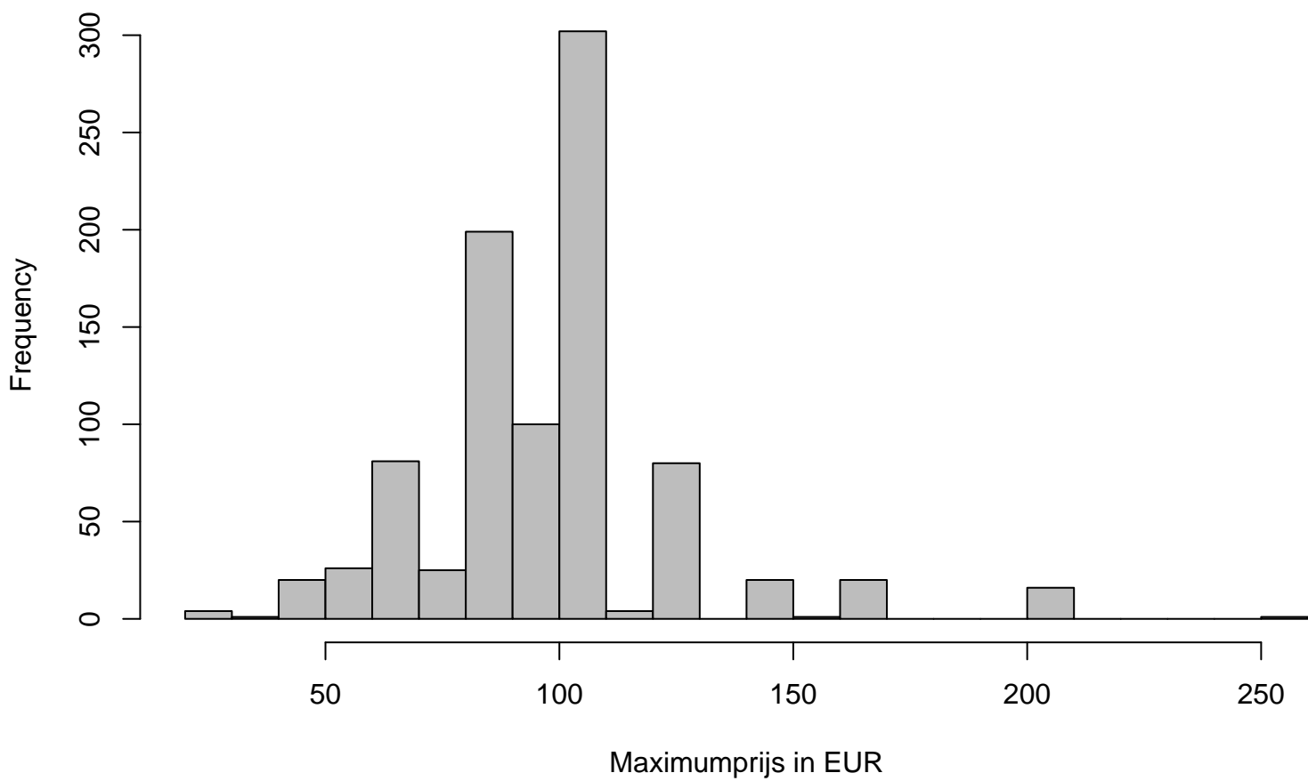
Histogram Maximumprijs TML
