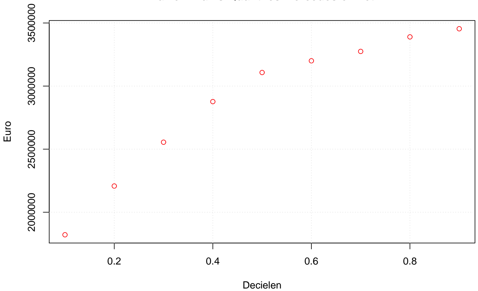
Harrell-Davis Quantiles Mercedes omzet
