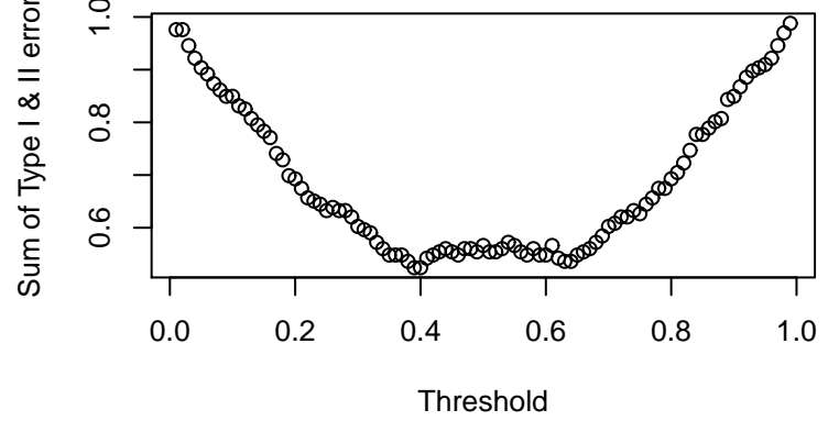
(1-Sens.) + (1-Spec.)
