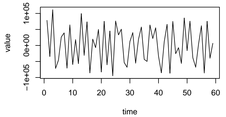
d=1, D=0
