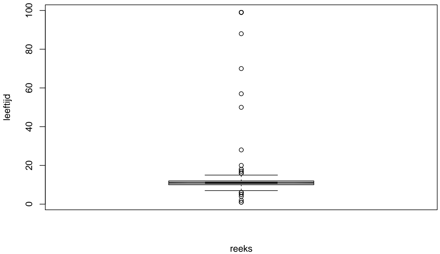
Boxplot studio 100 maximumleeftijd 2005
