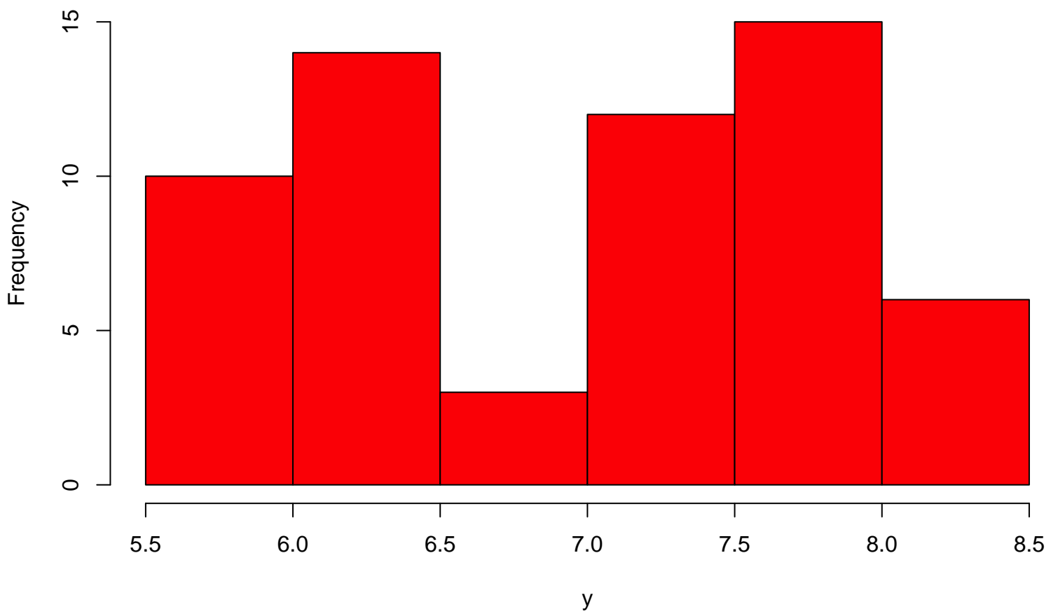
Histogram of y
