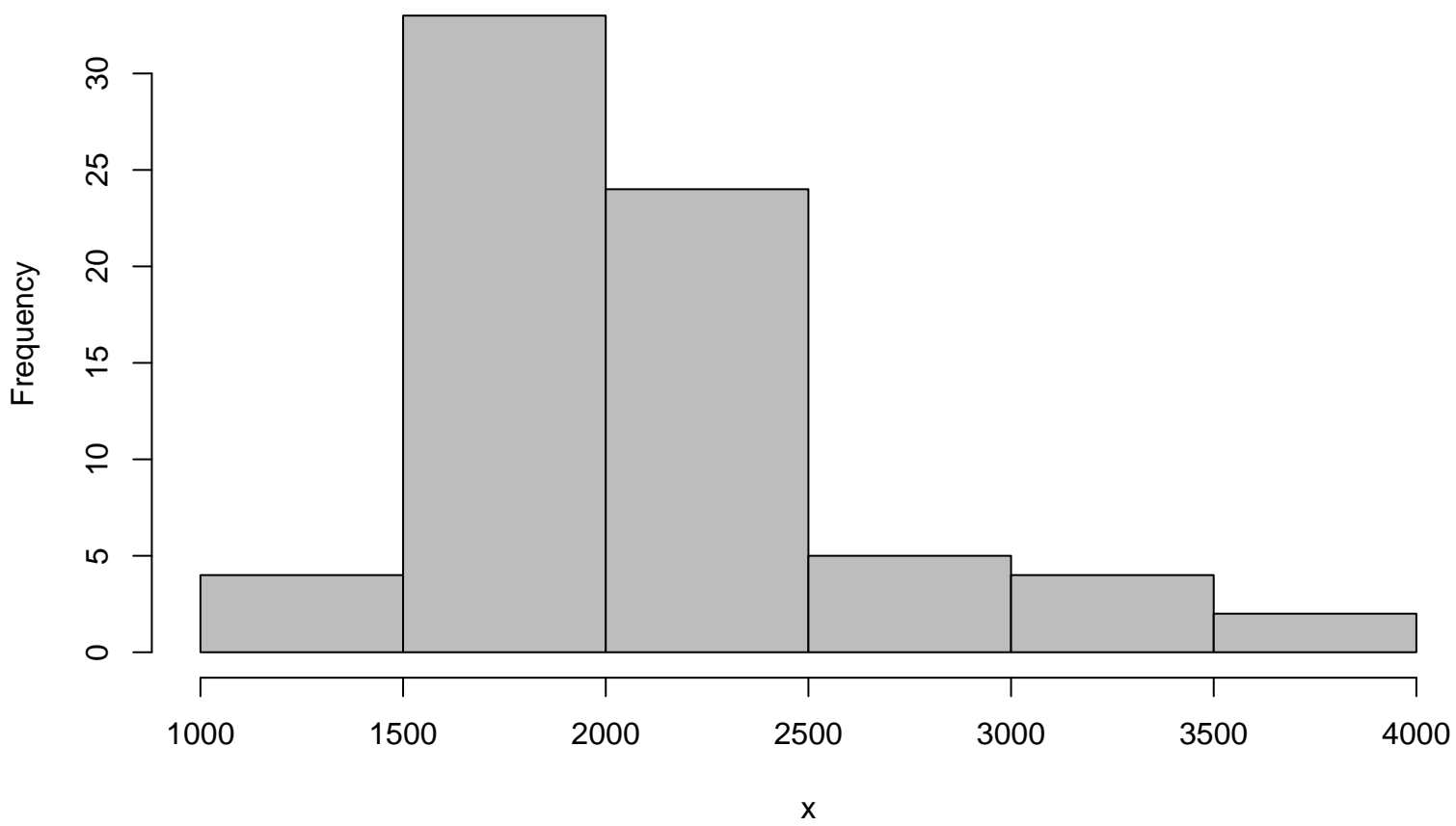
Histogram gebouwen 2009 –2014
