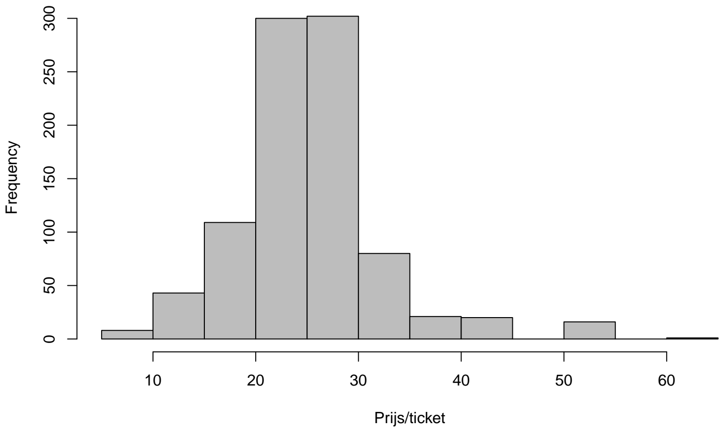
Histogram 12klassen
