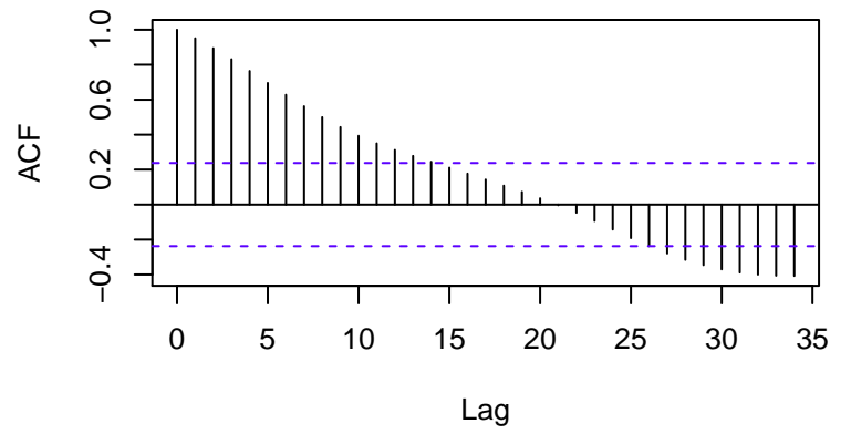
Trend
