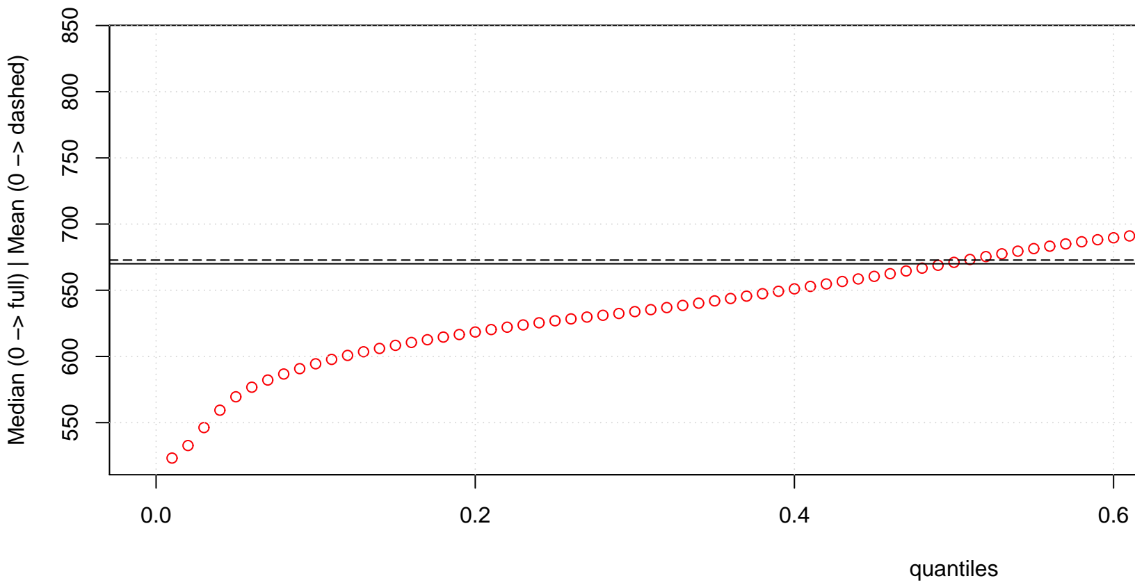
Harrell–Davis Quantiles
