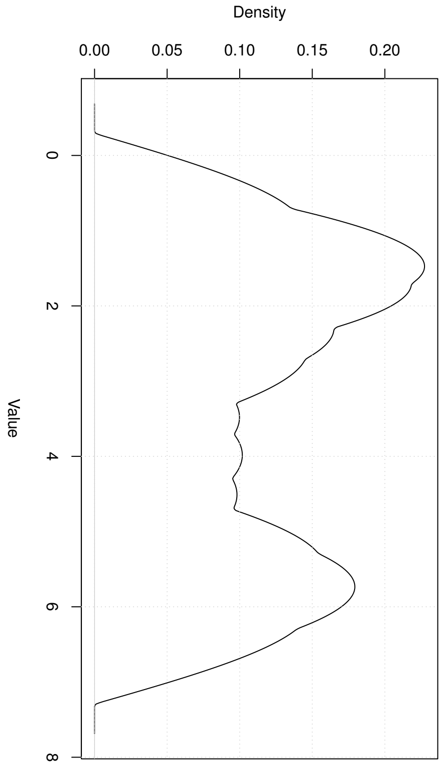
Opticosine Kernel
