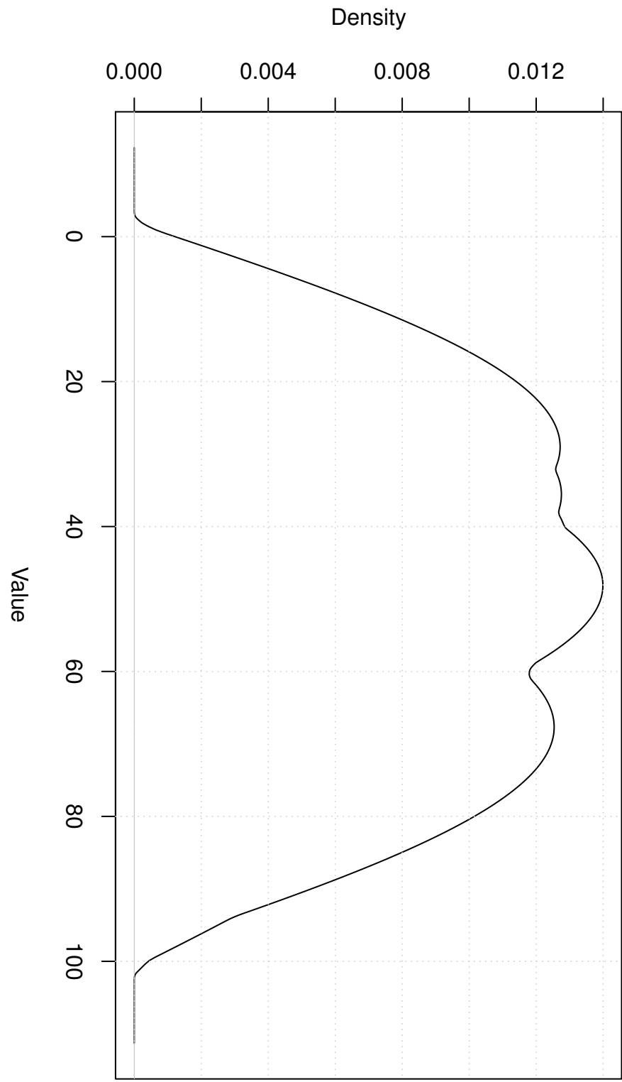
Opticosine Kernel
