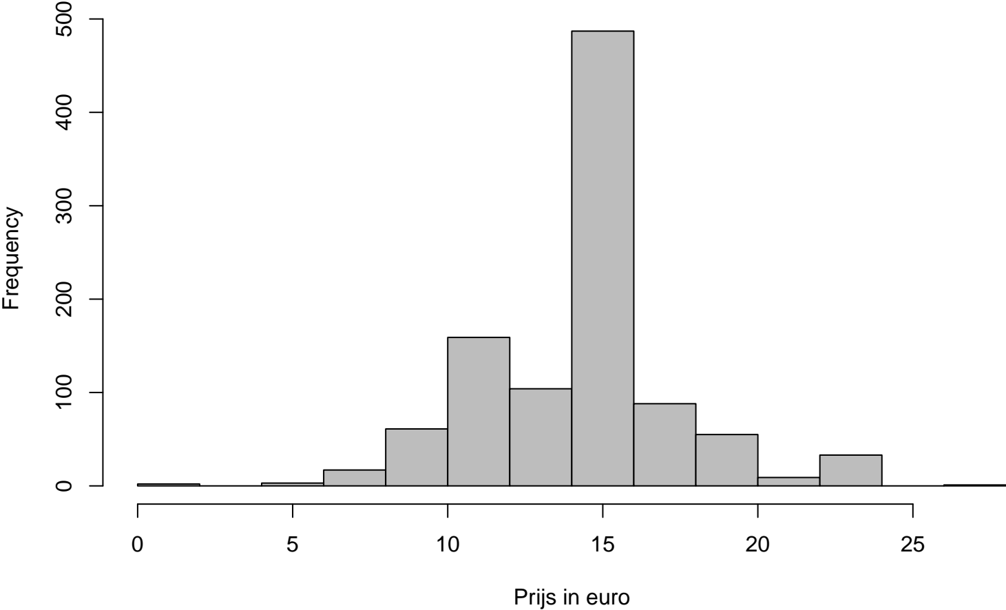
Histogram Maximumprijs Bioscooptickets
