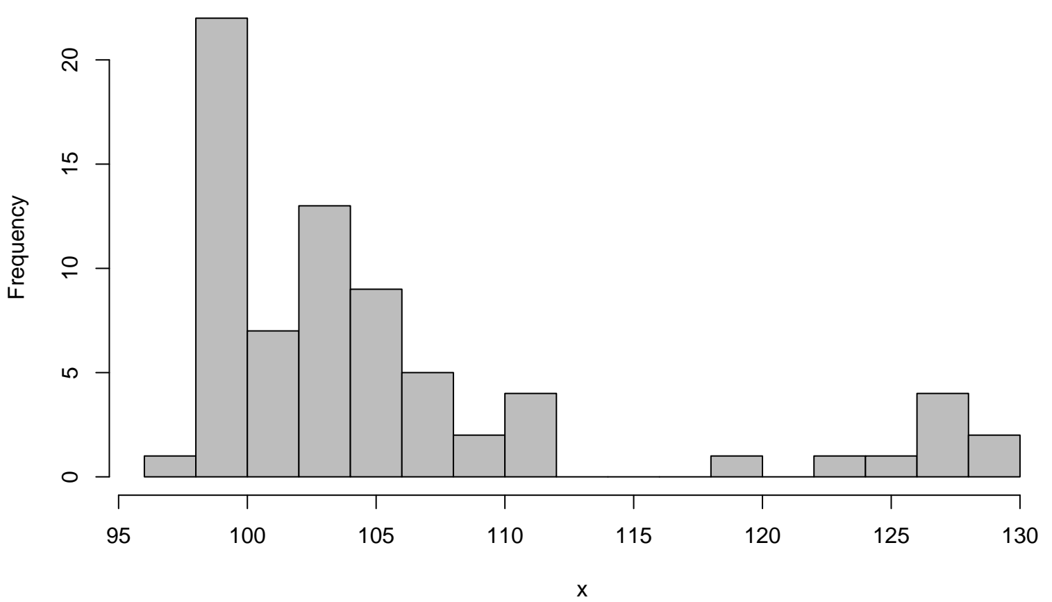
Histogram 12 klassen
