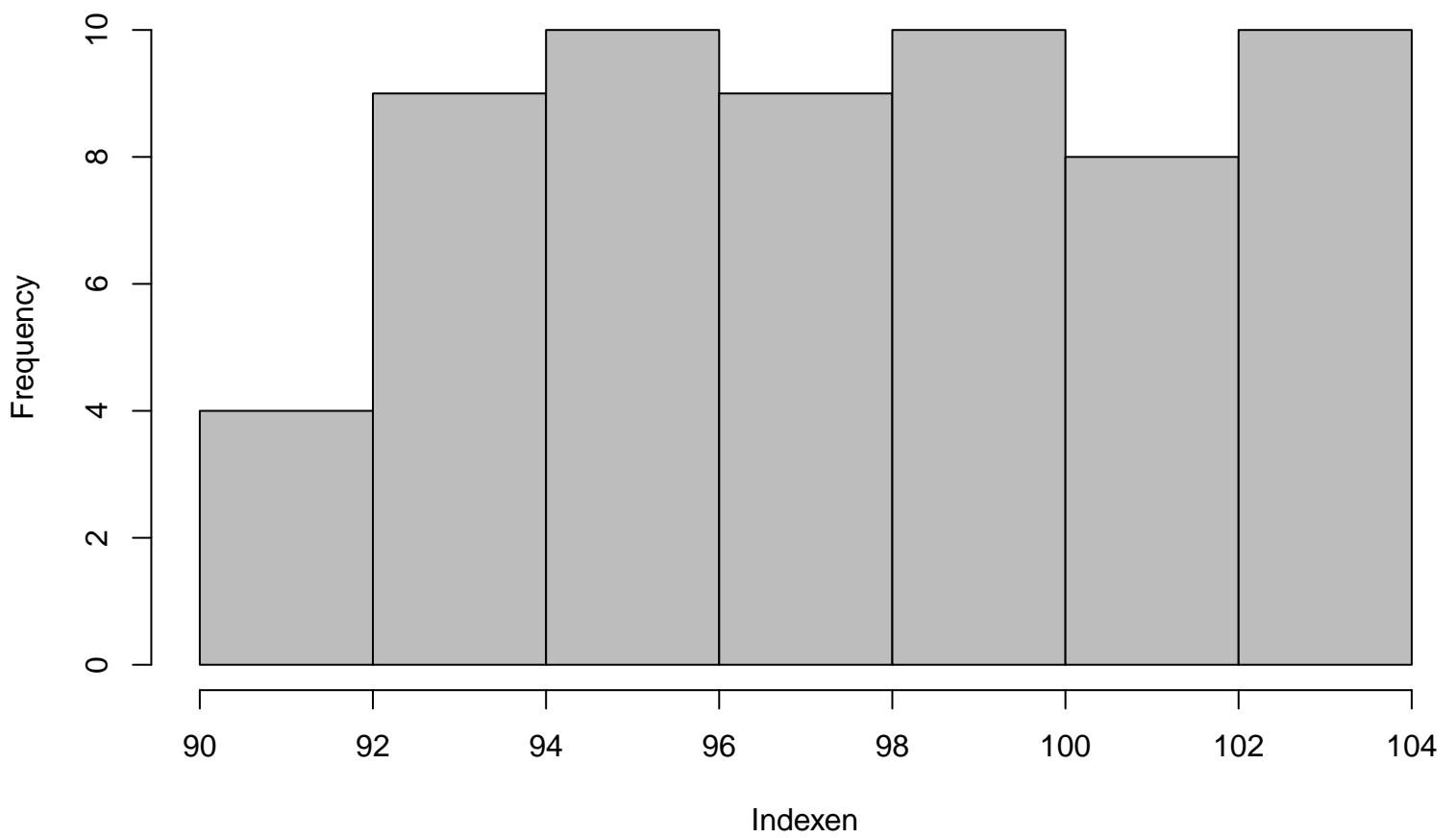
Histogram eigen cijferreeks
