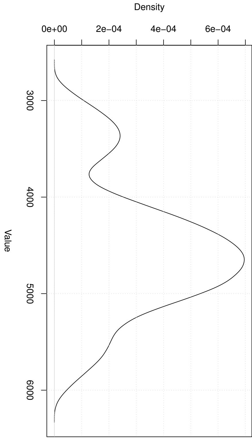
Cosine Kernel
