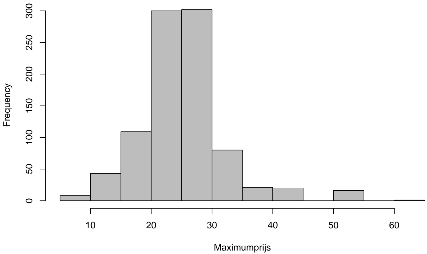
Histogram maximumprijs 2014
