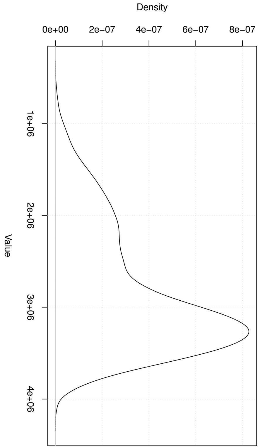
Cosine Kernel
