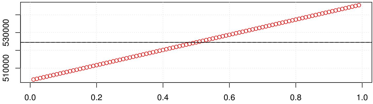
Harrell–Davis Quantiles
