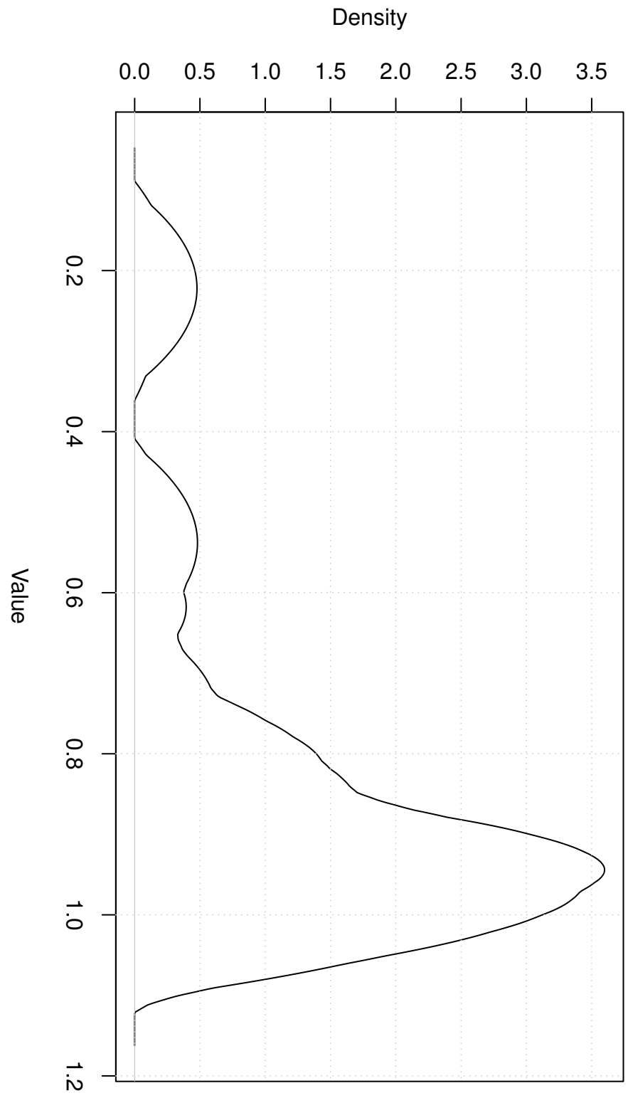
Epanechnikov Kernel
