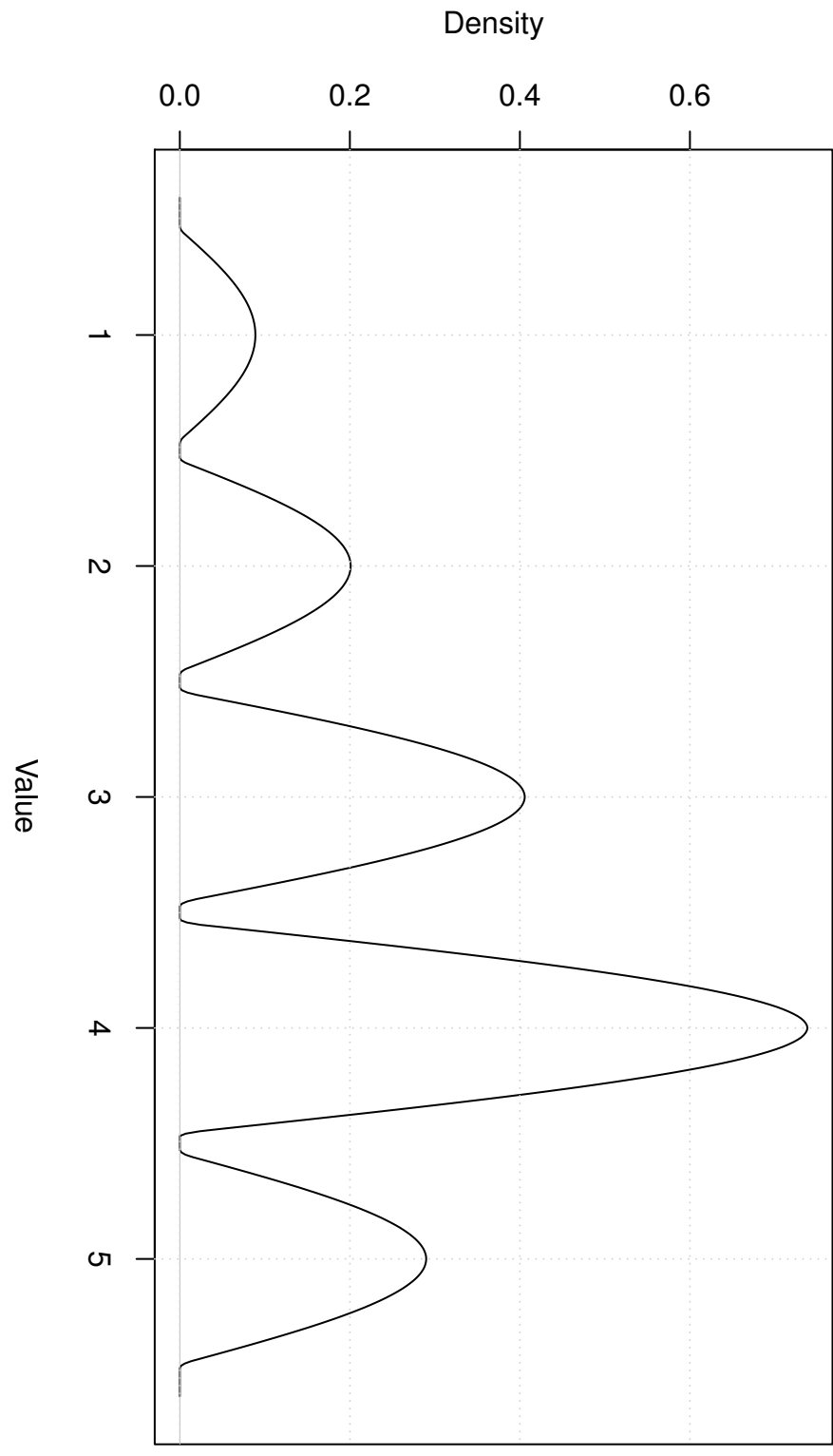
Opticosine Kernel
