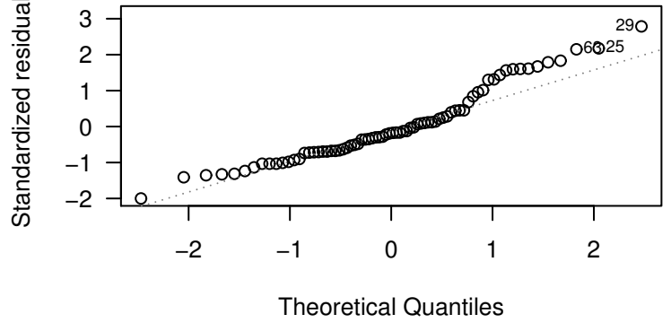
Normal Q-Q
