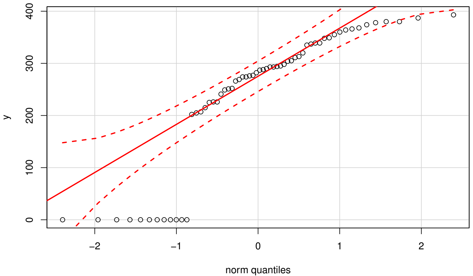
QQplot of variable y
