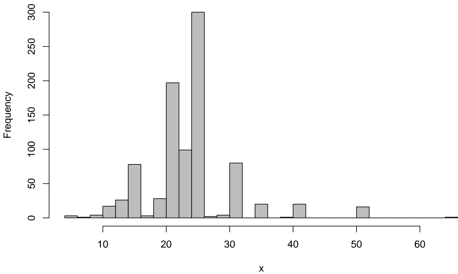
Histogram maximumprijzen show 2014
