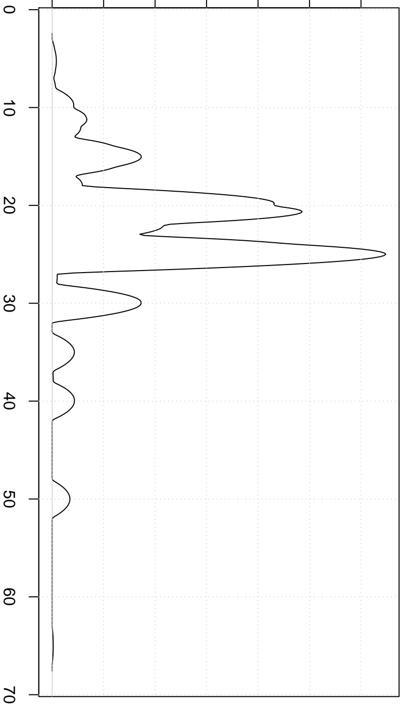
Epanechnikov Kernel
