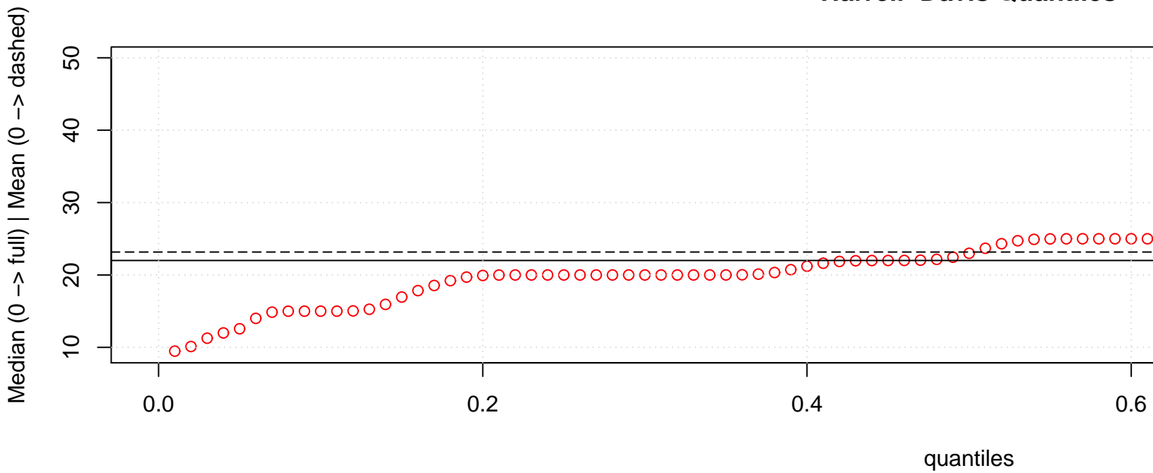
Harrell–Davis Quantiles
