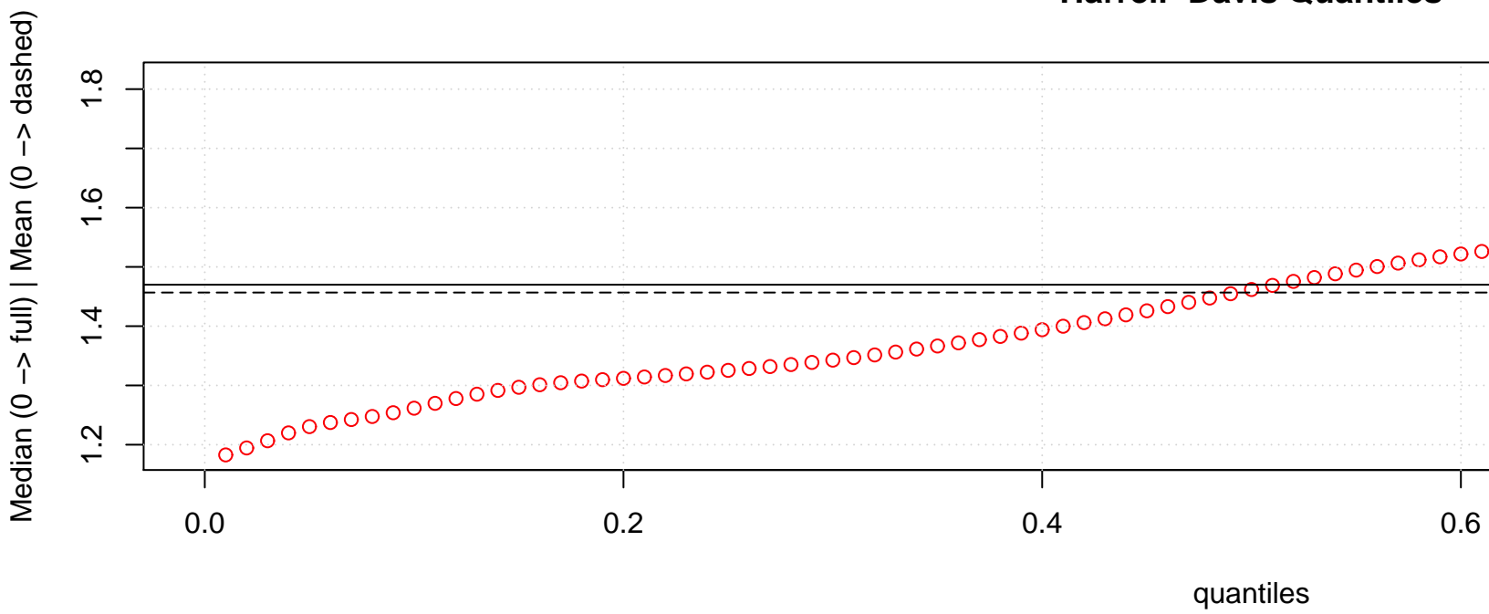
Harrell–Davis Quantiles
