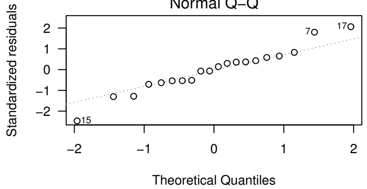
Normal Q-Q
